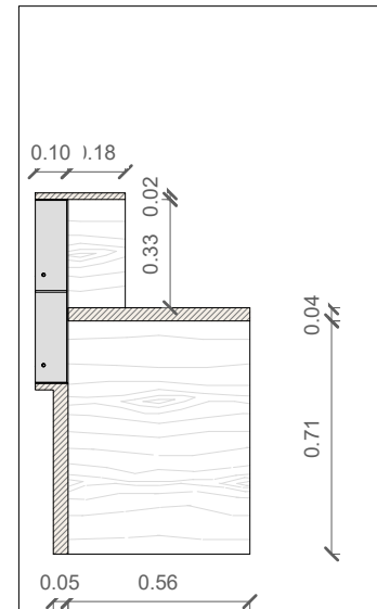
4 | ΤΑΜΕΙΟ ΤΟΜΗ 1 1 : 25
