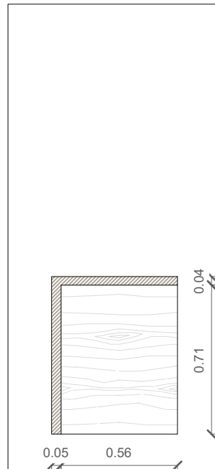
5 | ΤΑΜΕΙΟ ΤΟΜΗ 2 1 : 25
