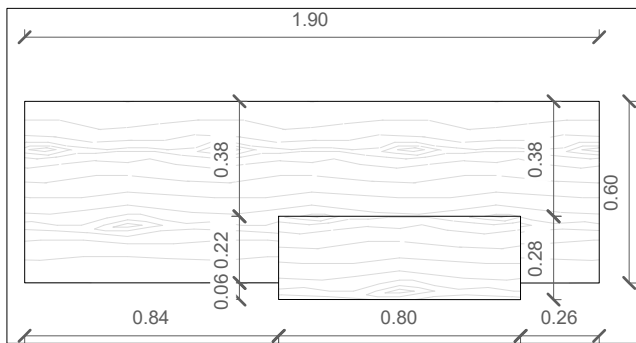
2 | ΤΑΜΕΙΟ ΚΑΤΟΨΗ 1 : 25
